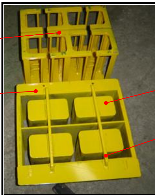
PRESSaBLOCS – MOULE 15-C et POINÇONS correspondants
